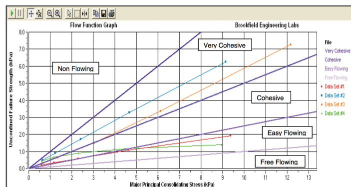
График функции текучести (кувета 230 см³)
