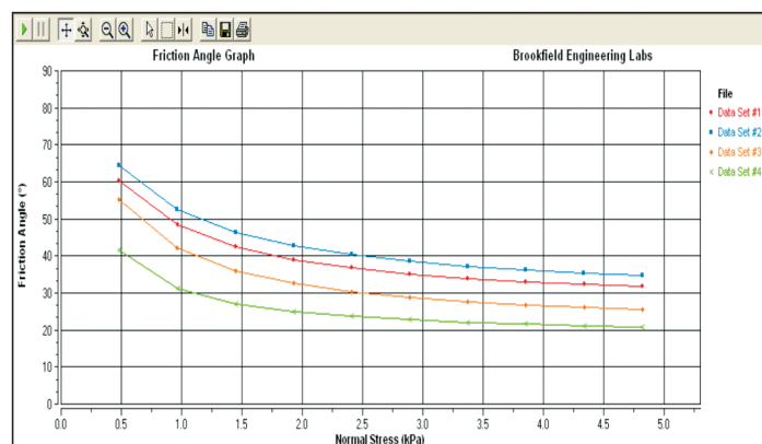
График угла пристеночной адгезии (кувета 230 см³)
