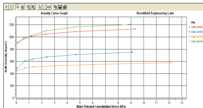
График насыпной плотности (кувета 230 см³)
