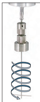
Вискозиметр DV1MRV (стр. 12) Стойка спирального движения Helipath, модель D (стр. 39)
